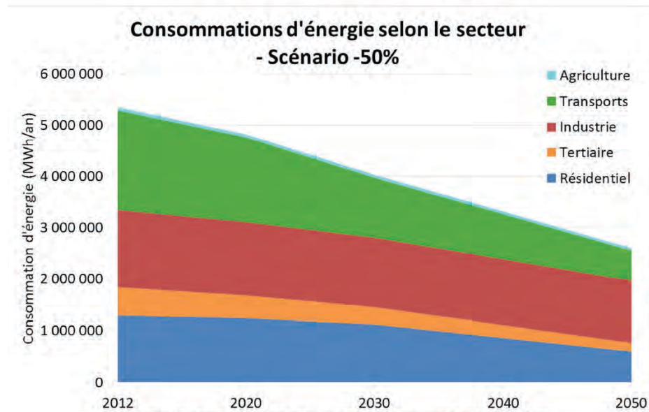
Figure 28 : Consommation d'énergie selon le secteur – Scénario -50%
